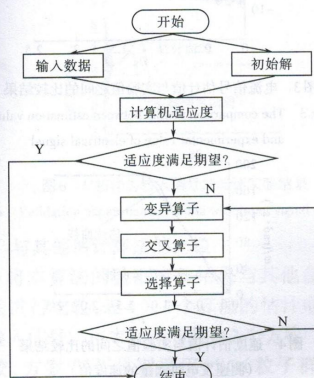
图1 改进的遗传算法流程图
