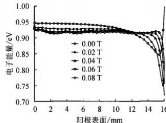
图9 不同纵向磁场下阳极表面电子温度
