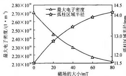
图8 磁场大小与最大电子密度/弧柱区半径关系
