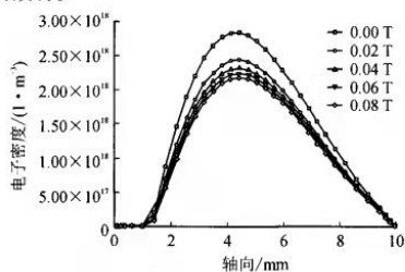
图7 不同纵向磁场下轴向电子密度分布
