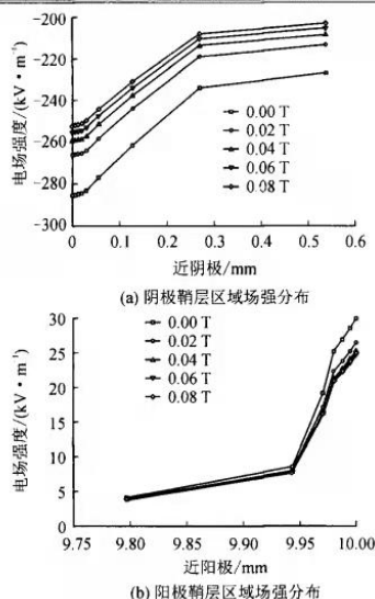
图6 不同纵向磁场下近阴极与近阳极电场强度分布
