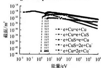
图2 Cu的碰撞截面
